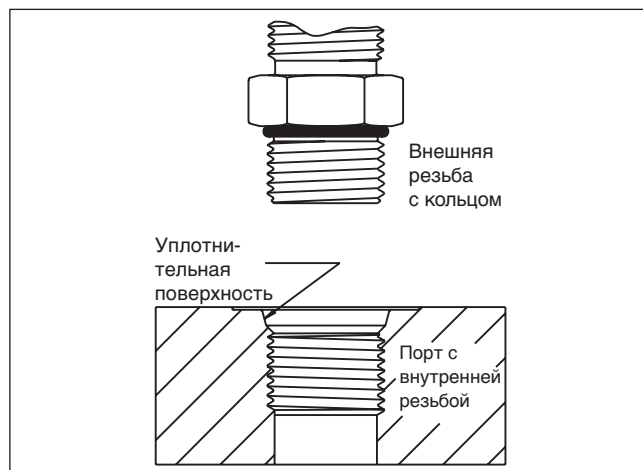
Рис. 5 – штуцер UNF
