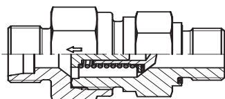
Конус EO 24° / Наружная метрическая резьба – Уплотнитель ED (ISO 9974)
