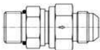
Наружная резьба UN/UNF – Уплотн. кольцо (ISO 11926) / Triple-Lok® 37°
