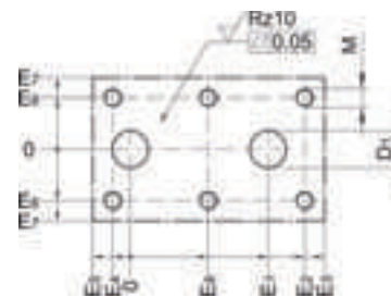
Шаблон для сверления
