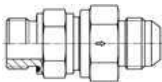
Наружная резьба BSPP – Уплотнитель ED (ISO 1179) / Triple-Lok® 37°
