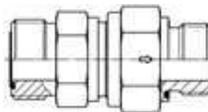
O-Lok® ORFS / Наружная резьба BSPP – Уплотнитель ED (ISO 1179)
