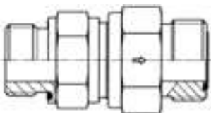
Наружная метрическая резьба – Уплотнитель ED (ISO 9974) / O-Lok® ORFS
