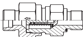
Конус EO 24° / Наружная резьба BSPP – Уплотнитель ED (ISO 1179)
