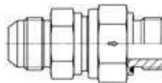
Triple-Lok® 37° / Наружная метрическая резьба – Уплотнитель ED (ISO 9974)
