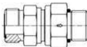
O-Lok® ORFS / Наружная резьба UN/UNF– Уплотн. кольцо (ISO 11926)
