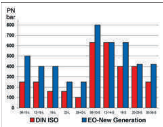
Номинальное давление
