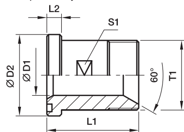
Поверхность уплотнительного кольца
