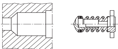
Внутренние части обратного клапана
