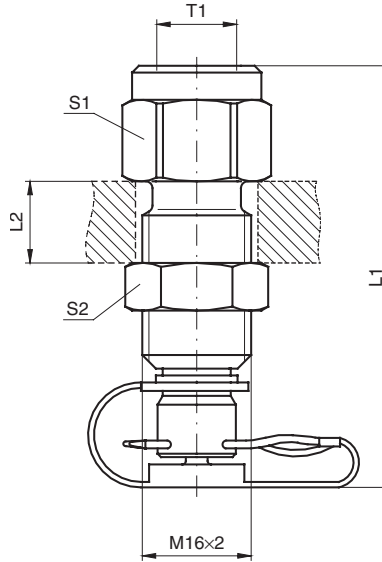
Фитинг под манометр: MAV-MA1
