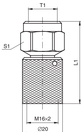
Фитинг для прямого подключения манометра: MAVMD...MA3
