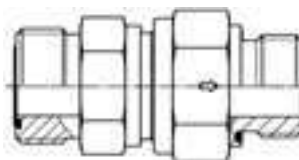
O-Lok® ORFS / Наружная метрическая резьба – Уплотнитель ED (ISO 9974)
