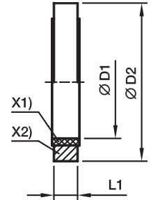
X1) Уплотнение PTFE X2) Опорное кольцо (Нерж. сталь)
