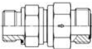
Наружная резьба BSPP – Уплотнитель ED (ISO 1179) / O-Lok® ORFS
