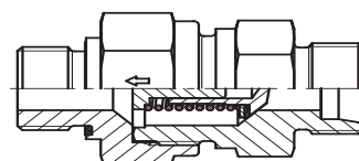
Наружная резьба BSPP – Уплотнитель ED (ISO 1179) / Конус EO 24°
