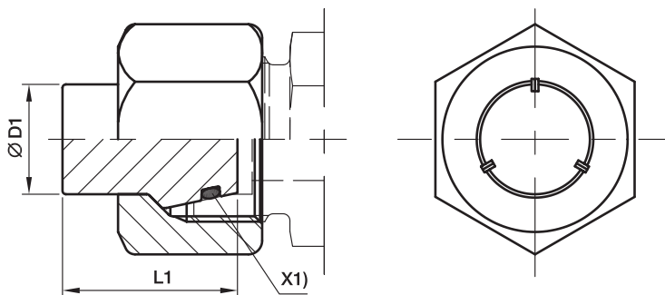
X1) Уплотн. кольцо OR
