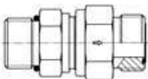
Наружная резьба UN/UNF– Уплотн. кольцо (ISO 11926) / O-Lok® ORFS
