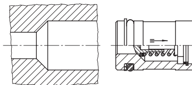
Картридж обратного клапана
