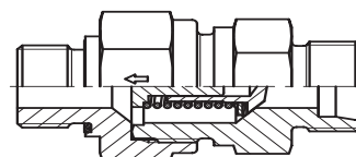
Наружная метрическая резьба – Уплотнитель ED (ISO 9974) / Конус EO 24°
