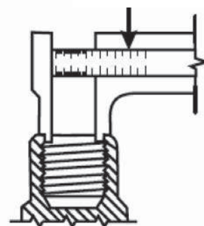
Внутренний диаметр резьбы
