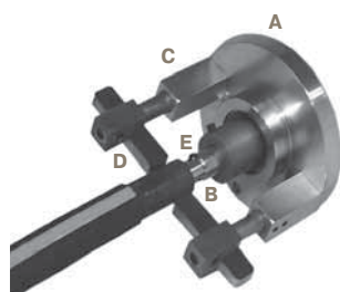
Инструмент для окорки А: Держатель оснастки в сборе В: Оправка для внутренней окорки С: Держатель для ножа наружной окорки Д: Нож для наружной окорки Е: Нож для внутренней окорки
